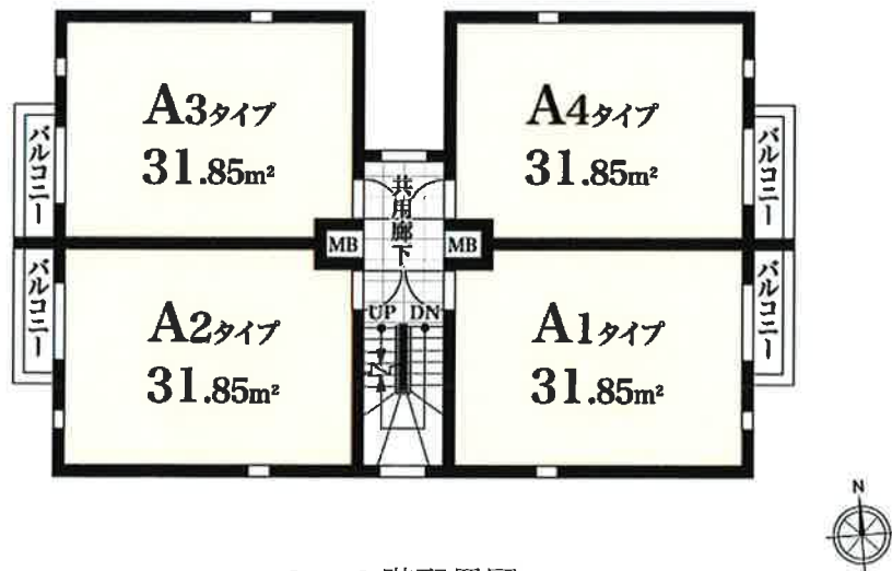
2・3階配置図
